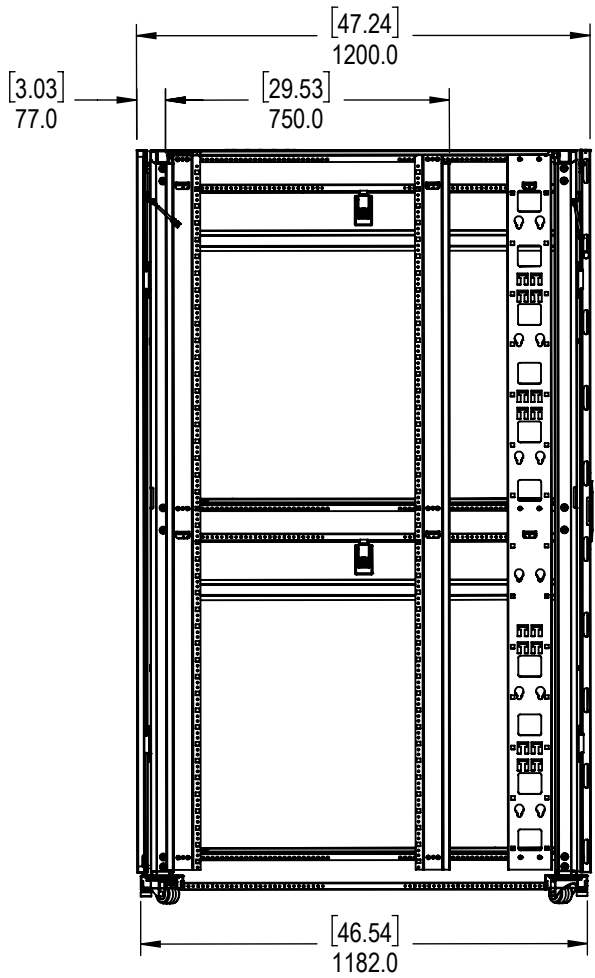
SECTION A-A
