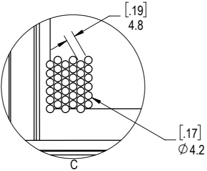
C SCALE 1 : 2
