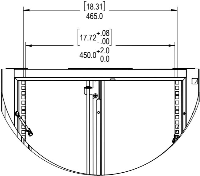
B SCALE 1 : 7
